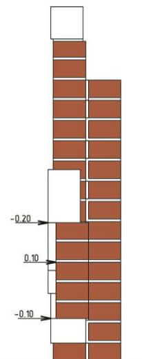
Разрез 1-1 М 1:15
